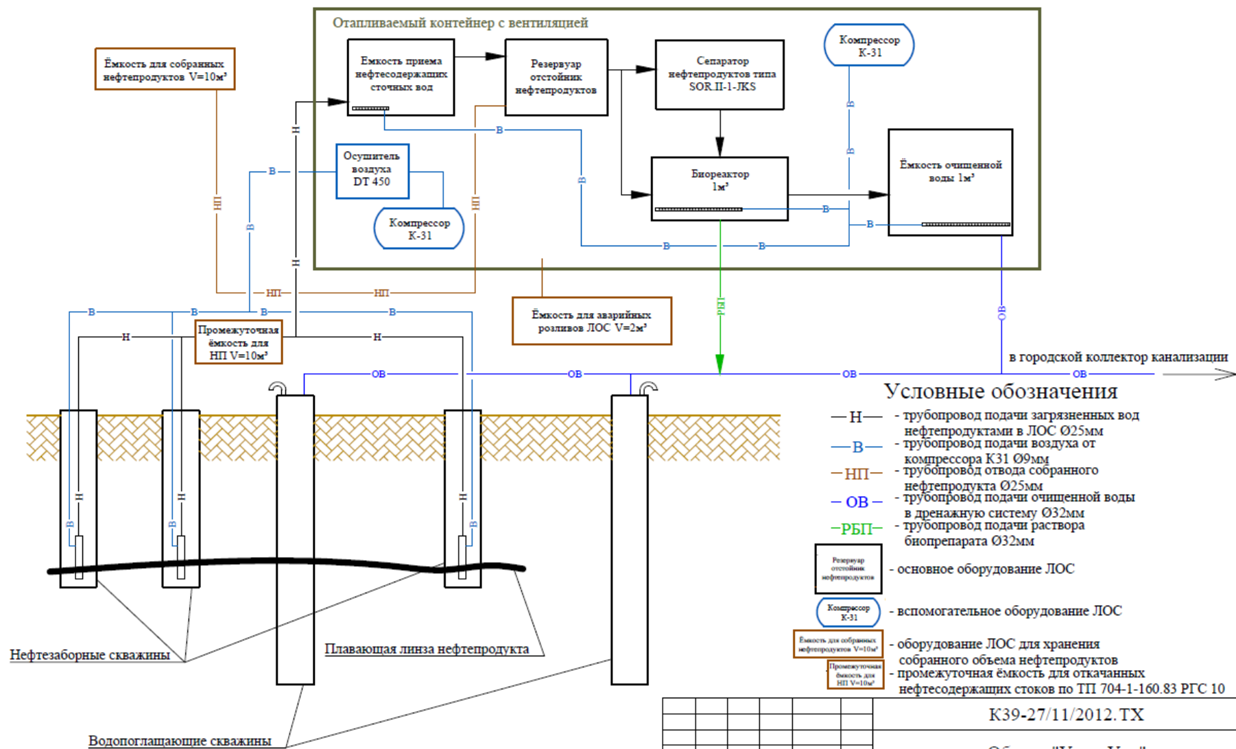
Схема ликвидации линзы нефтепродуктов
