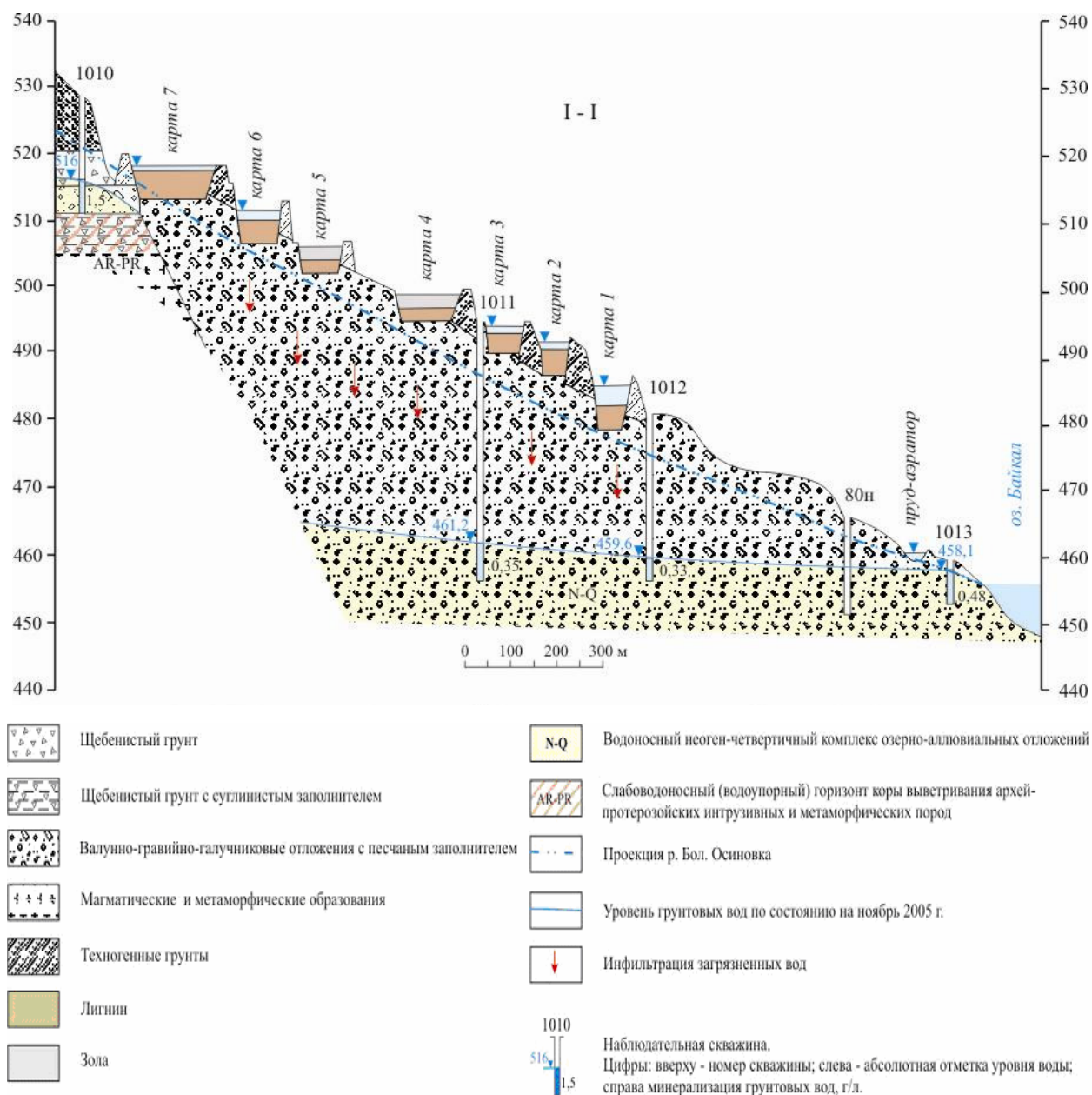
Рис. 1.3.1.5. Геолого-гидрогеологический разрез по участку накопителей лигнина и золы в прибрежной зоне Байкала на Солзанском участке
