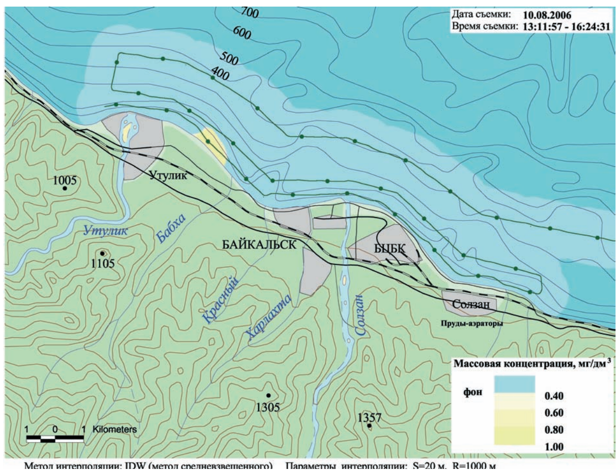
Рис. 1.3.1.8 Площадная съемка комплексом «Акватория-Байкал». Хлорид-ионы
